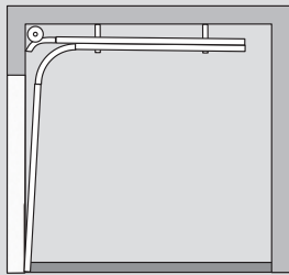
Nadproże Standard STH (sprężyny skrętne z przodu)
