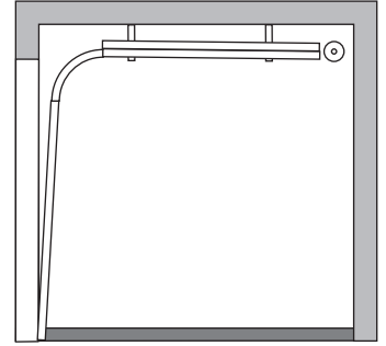
LHR niskie ze sprężynami z tyłu
