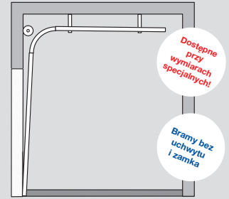
Nadproże Wysokie H (sprężyny skrętne z przodu)
