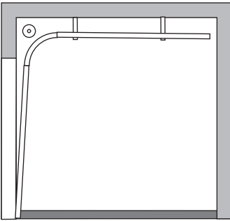
FTR Standardowe wzdłuż konstrukcji dachu
